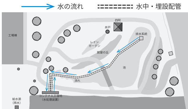
図 1 鉛直流式人工湿地を利用した池の水質改善
