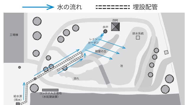
図 2 浸透水平流式人工湿地による雨水の浄化
